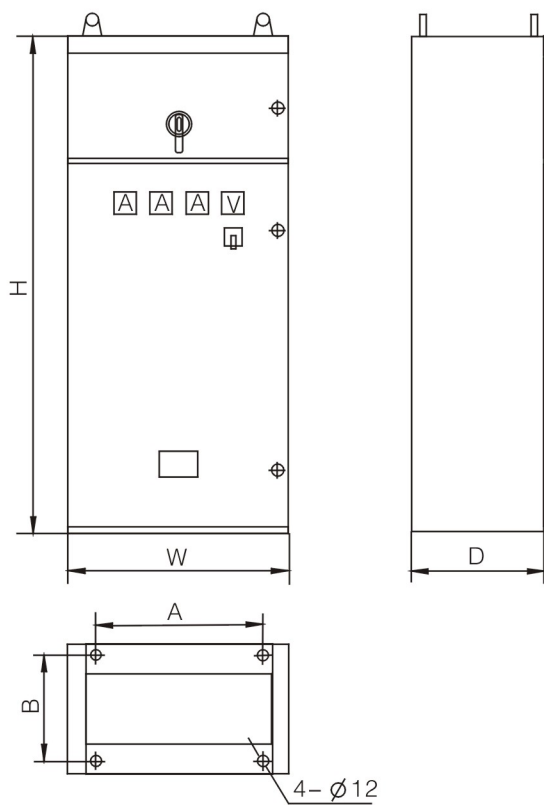
XL-21(G)型动力柜外形及安装尺寸图
